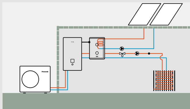
Serie Aquarea H e J: Serbatoio di accumulo con valvola solare e miscelatrice
