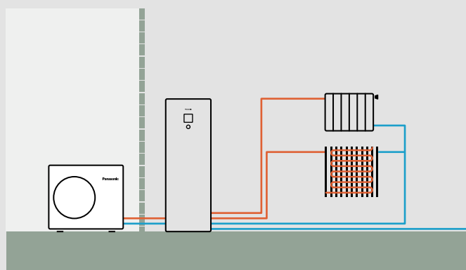
Aquarea All in One a 2 zone serie H e J: A 2 zone integrata, senza serbatoio di accumulo
