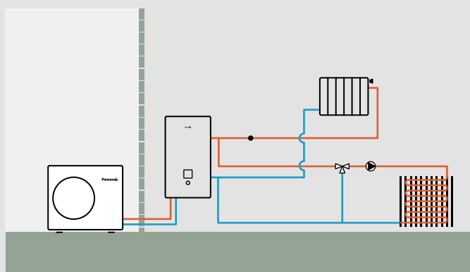
Serie Aquarea H e J: A 2 zone con kit esterno senza serbatoio di accumulo
