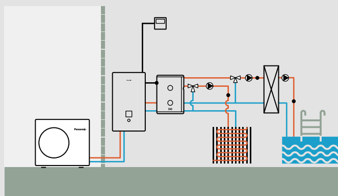
Serie Aquarea H e J: A 2 zone con kit esterno, serbatoio di accumulo e piscina
