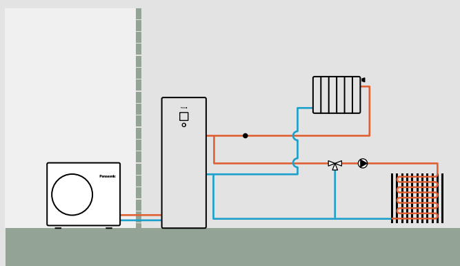
Aquarea All in One serie H e J: A 2 zone con kit esterno senza serbatoio di accumulo
