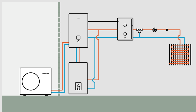
Serie Aquarea H e J: Bivalente con serbatoio di accumulo e valvola di miscelazione
